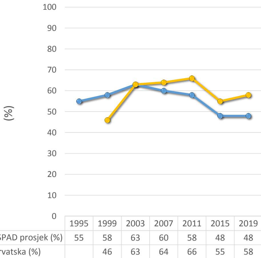
ESPAD prosjek i Hrvatska (trend 1995. – 2019.)
