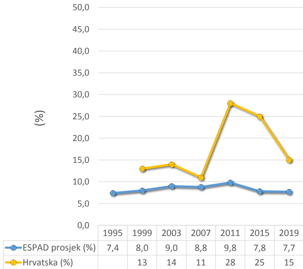
ESPAD prosjek i Hrvatska (trend 1995. – 2019.)
