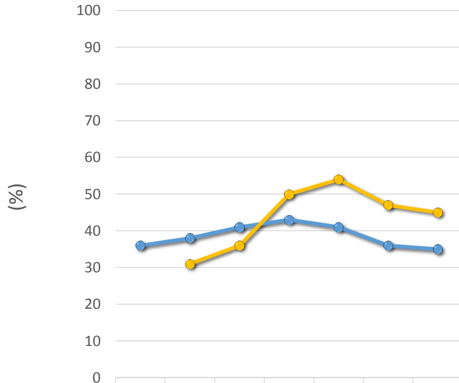
ESPAD prosjek i Hrvatska (trend 1995. – 2019.)
