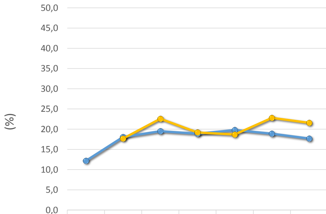
ESPAD prosjek i Hrvatska (trend 1995. – 2019.)
