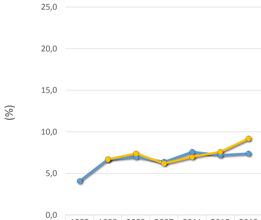
ESPAD prosjek i Hrvatska (trend 1995. – 2019.)
