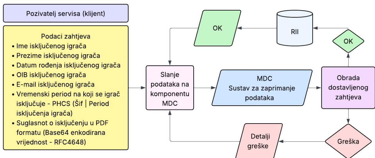
Schema pozivanja servisa za slanje podataka o isključenim igračima
