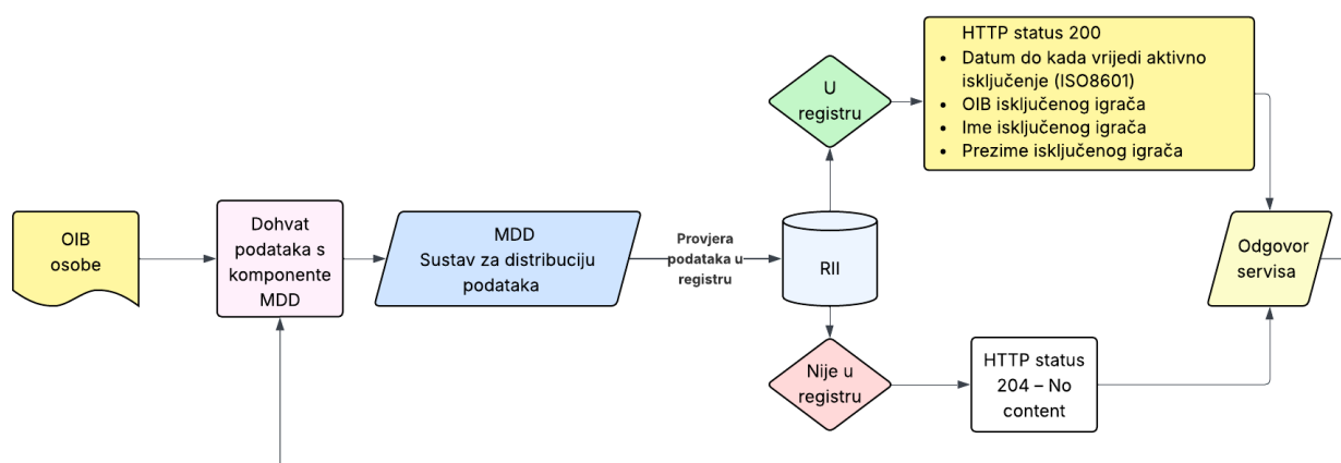
Schema pozivanja servisa za provjeru podataka o isključenim igračima
